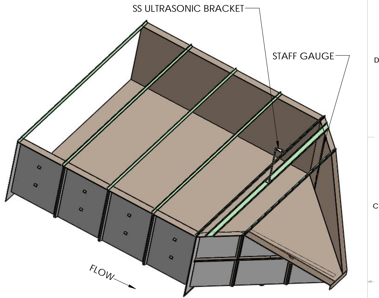
ISOMETRIC VIEW SCALE: 1:38
