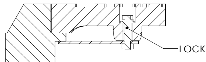
SECTION B-B SCALE 1 : 4
